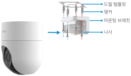
그림 1 천장 장착
