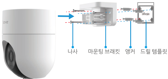
그림 2 벽 장착
